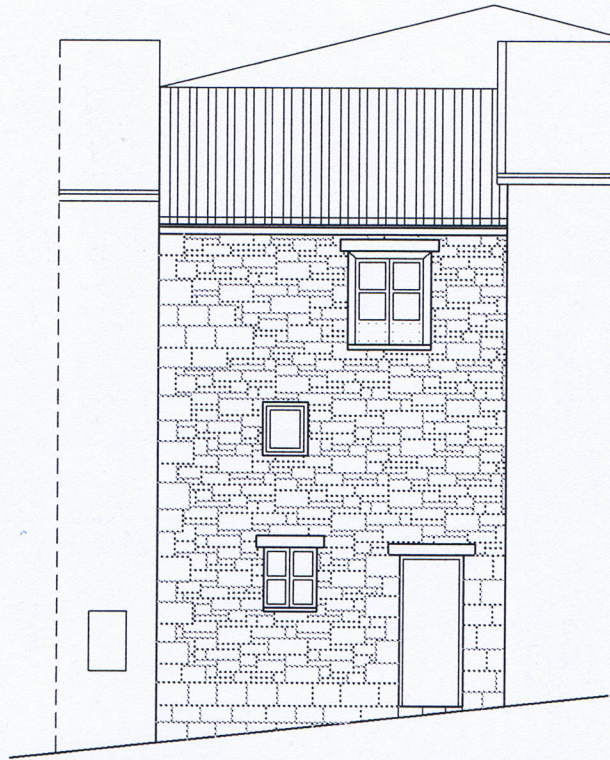
FACHADA LATERAL
